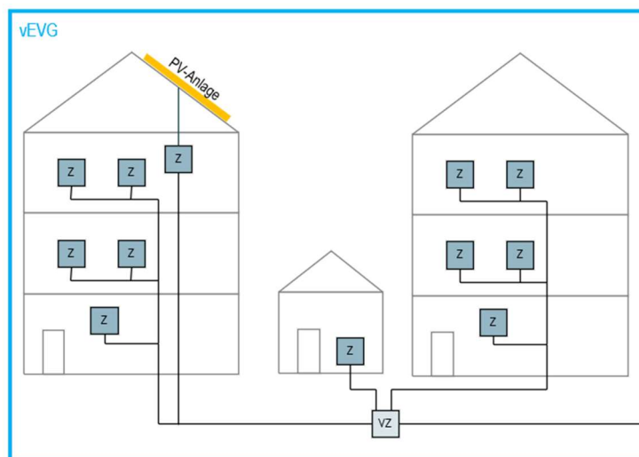
Physische Messungen (Z) und virtueller Überschussmesspunkt (VZ) am Verknüpfungspunkt (Bsp. Verteilkabine, Muffe, Trafostation) von der DKEK
