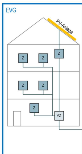
Physische Messungen (Z) und virtueller Überschussmesspunkt (VZ) am Anschlusspunkt
